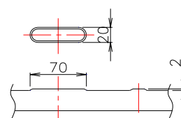
断面 Y-Y (滑り止め突起部)
